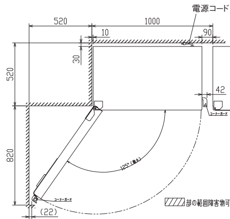
上面設置寸法図 (単位:mm)
